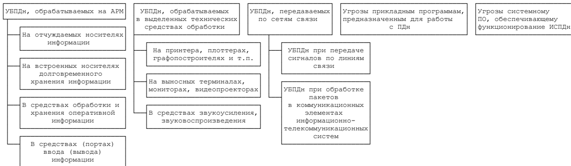
Рисунок 2. Классификация угроз безопасности персональных данных, обрабатываемых в информационных системах персональных данных
